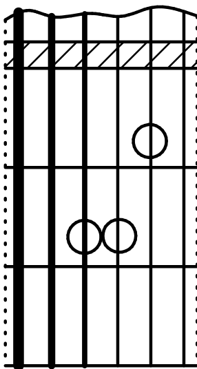
x Am
