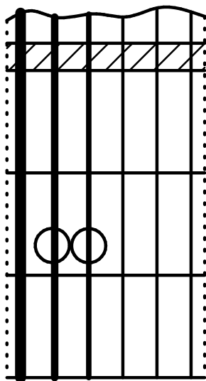
x Em
